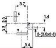
P.C.B. Land Pattern
