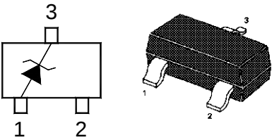
SOT-23
