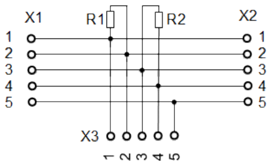
Рис. 1. Схема принципиальная ПР-ЗР
