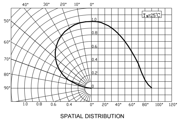
Radiation diagram 辐射图特性曲线
