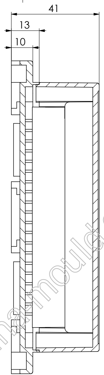
剖面 B-B
