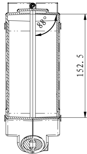
剖面A-A
