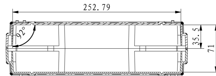
剖面B-B
