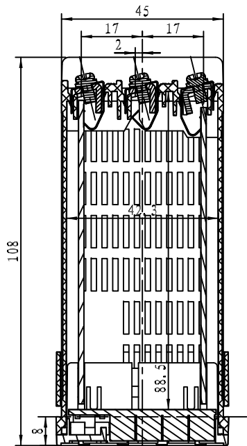
截面 A-A
