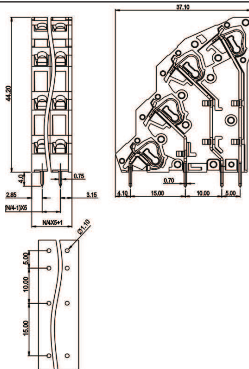
DG245H4-5.0 DG245H4-5.08
