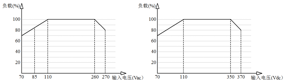
输入电压与负载特性曲线
