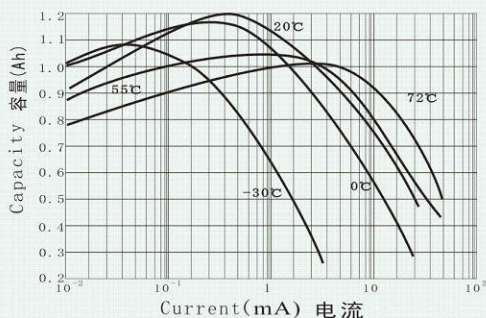
Capacity vs current 容量VS电流
