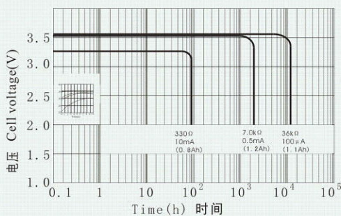
Discharge characteristics 放电特性 (25°C)
