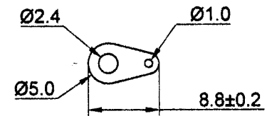
SOLDER LUG
