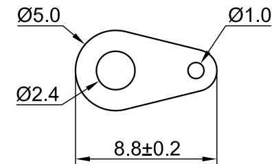
SOLDER LUG S=2
