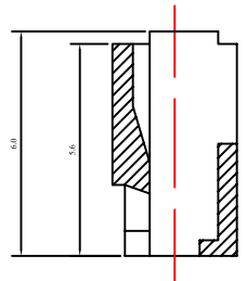
SEC.A-A
