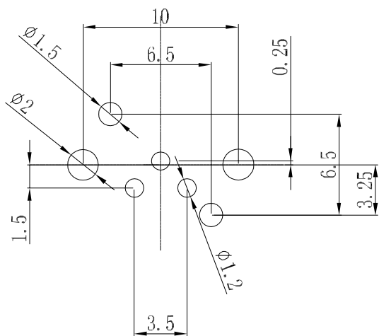
PBC板开板尺寸
