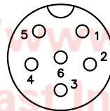
6 PIN(ø1.2 5A)
