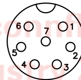
7 PIN(ø1.2 5A)
