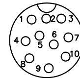
10 PIN( \phi 1.2 5A)
