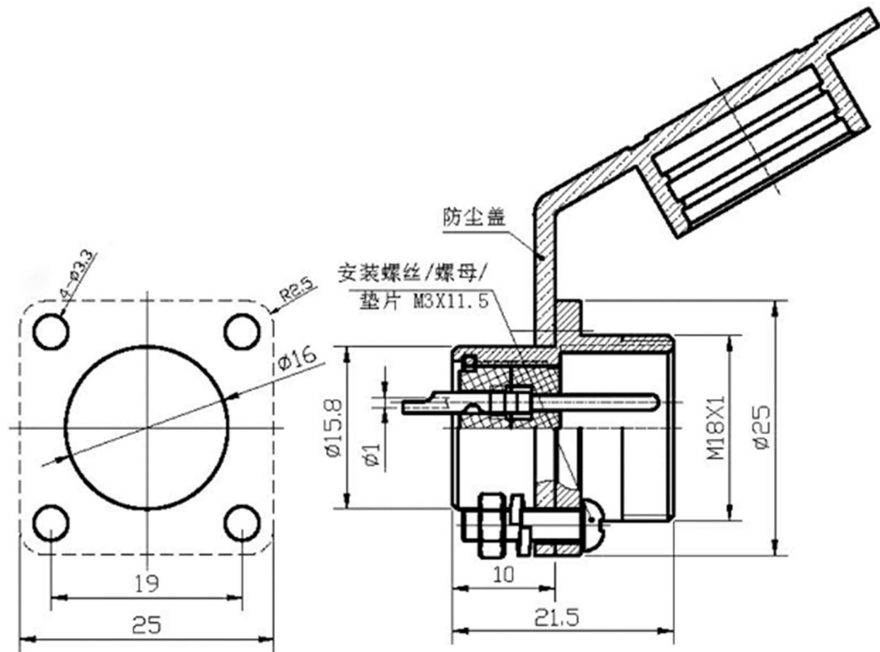
箱体开孔尺寸
