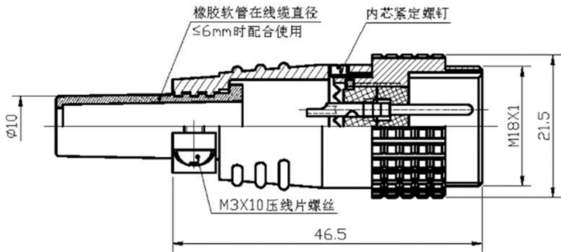
对接座 PLS16J_D
