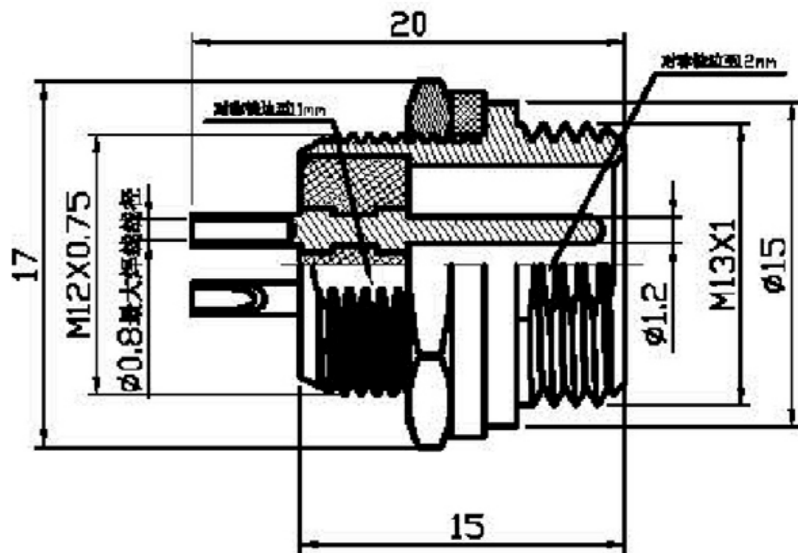
圆螺纹座 RS765-__B
