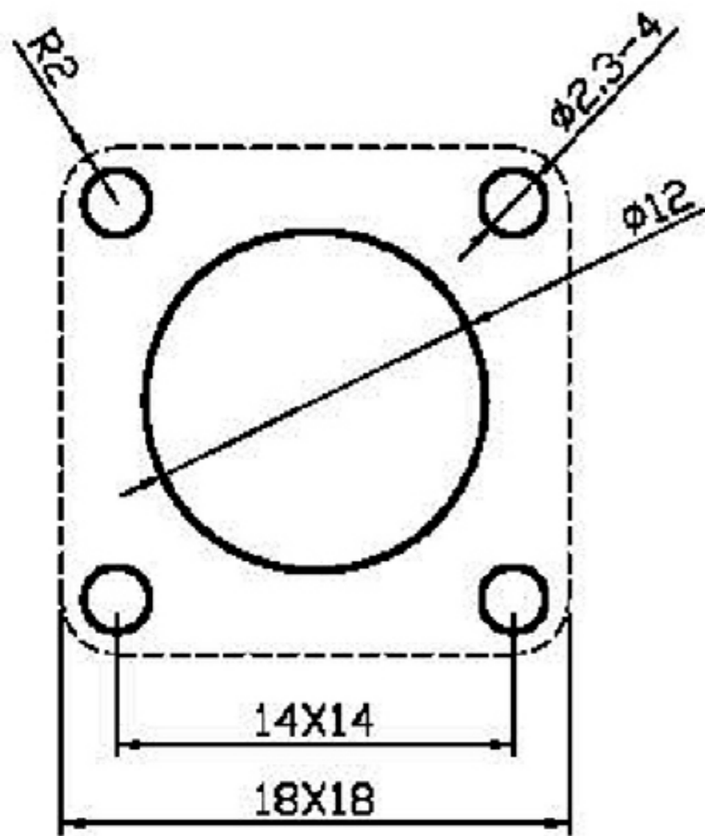
箱体开孔尺寸
