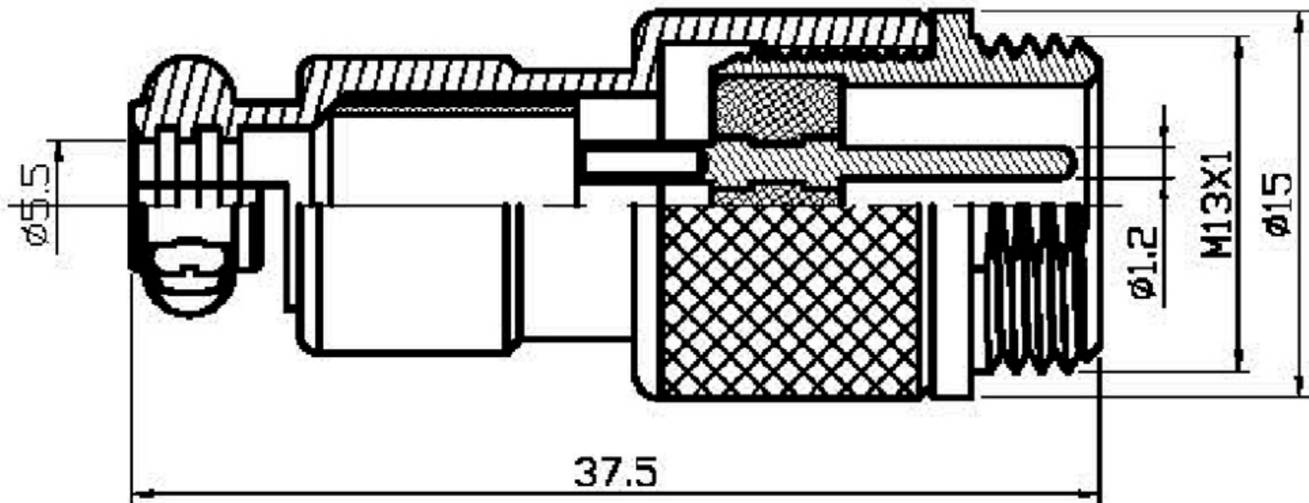
螺丝固定对接座 RS765-__K
