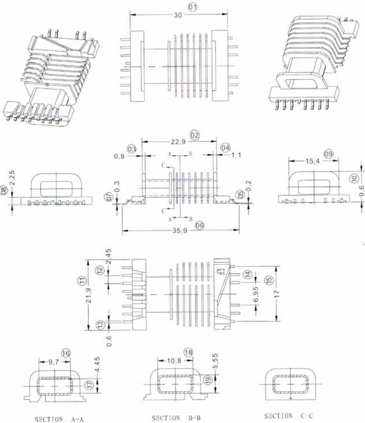
SECTION A-A
