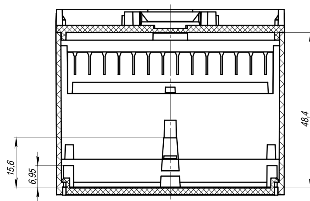
A-A (1.4:1)
