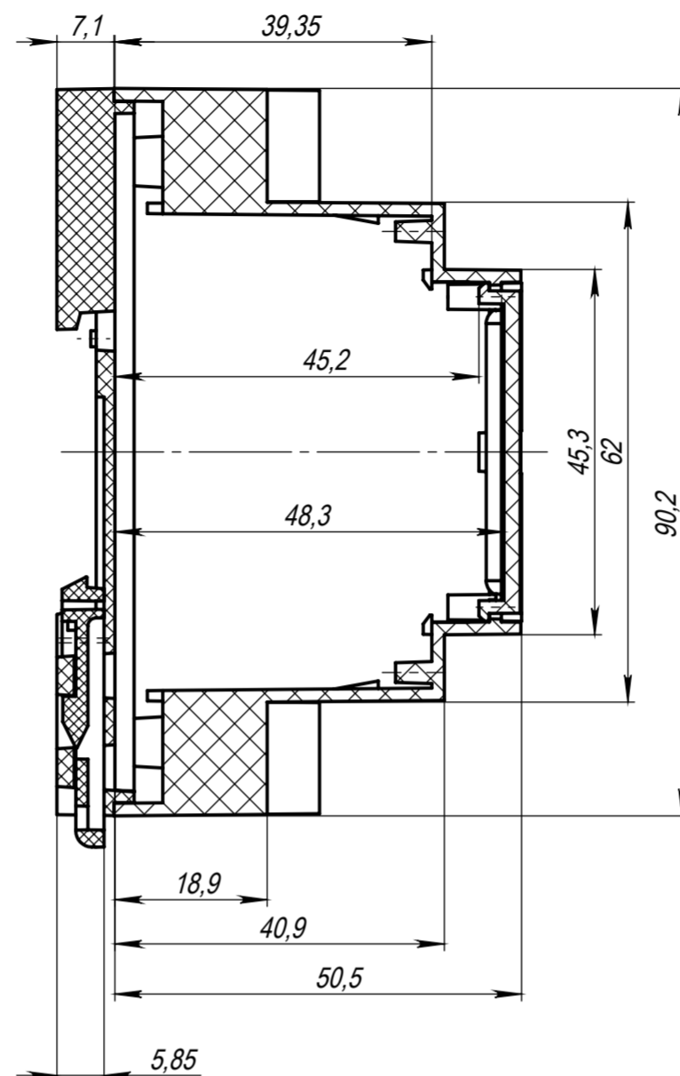
B-B (1.2 : 1)
