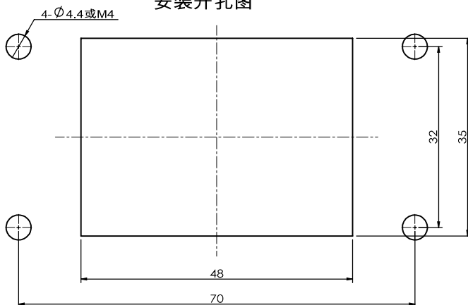
安装开孔图
