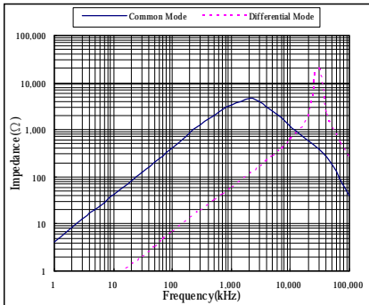
UF09V2/ UF09H2501YL□
