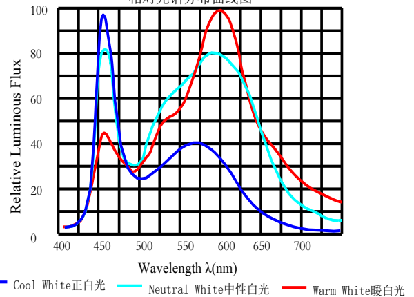
Wavelength Characteristics Ta=25°C 相对光谱分布曲线图
