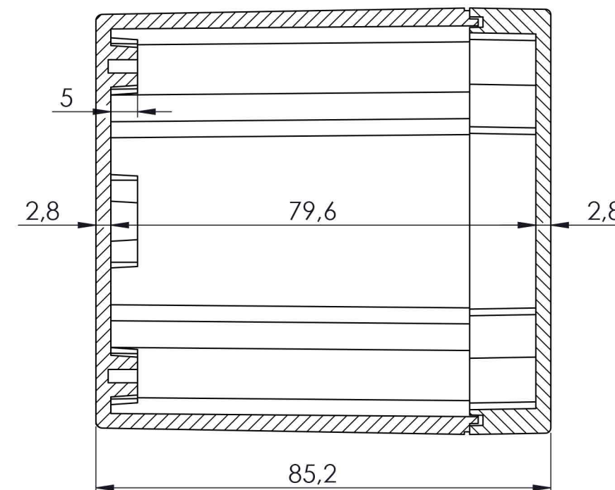
KESIT A-A
