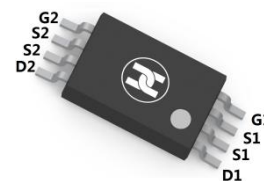
TSSOP-8
