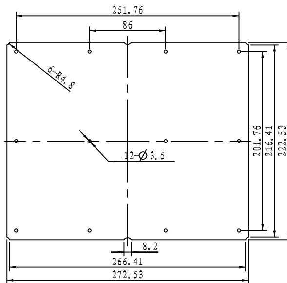
建议PCB尺寸
