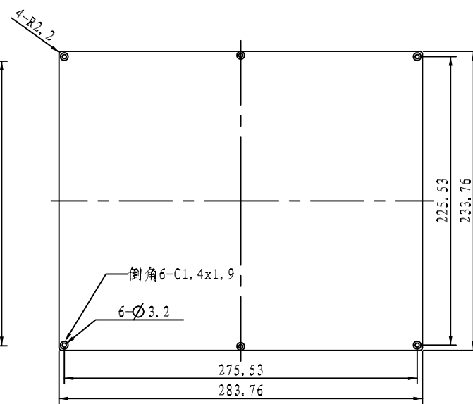
面板
