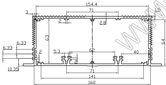
铝型材截面图
