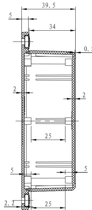
剖面 A-A
