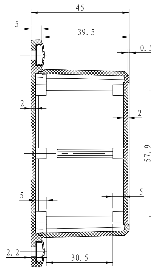
剖面 A-A
