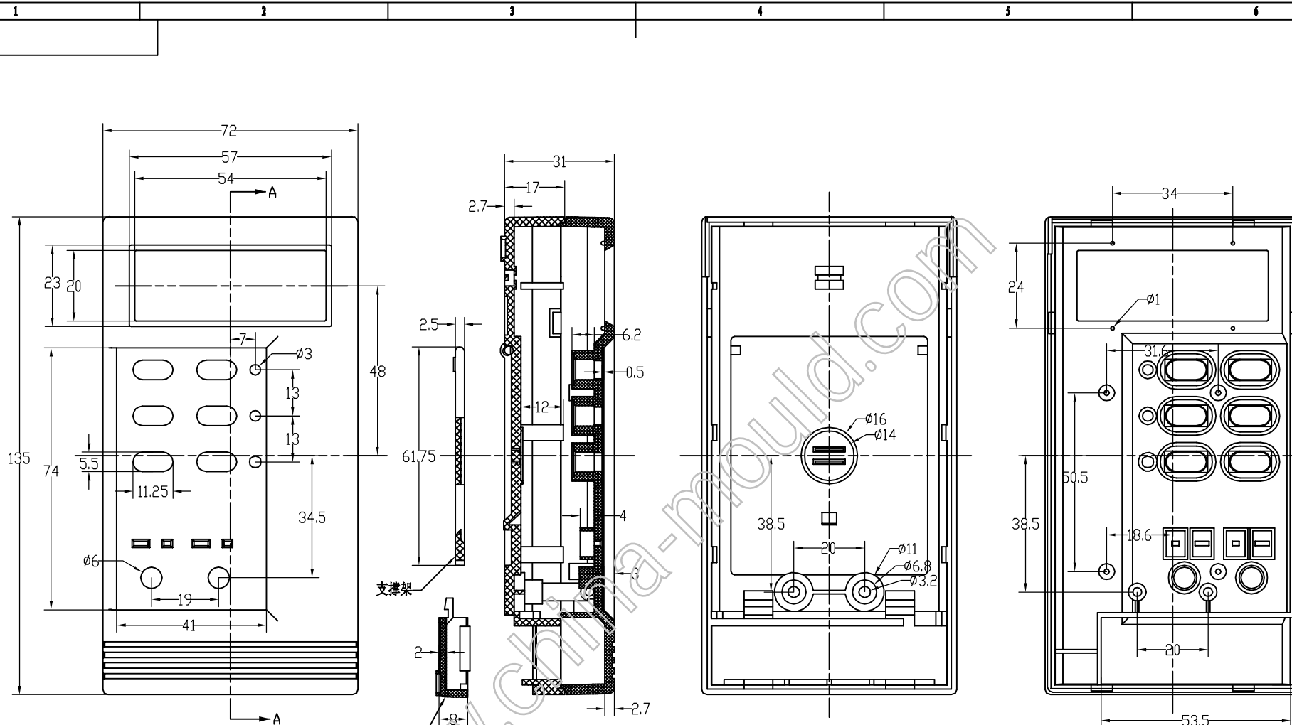
下盖正视图
