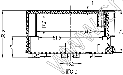
截面C-C
