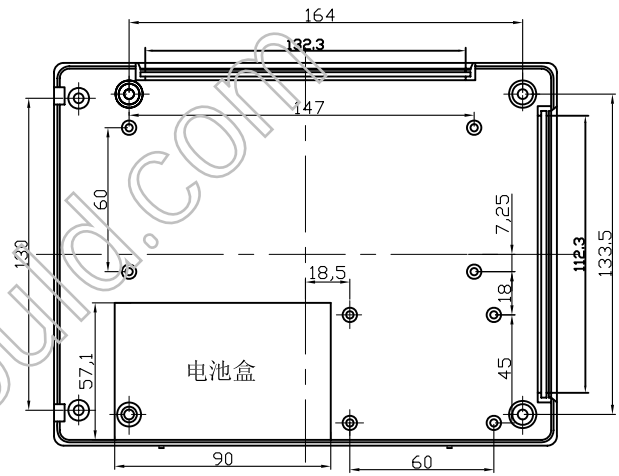
下盖正视图
