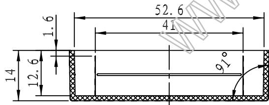
剖面 B-B
