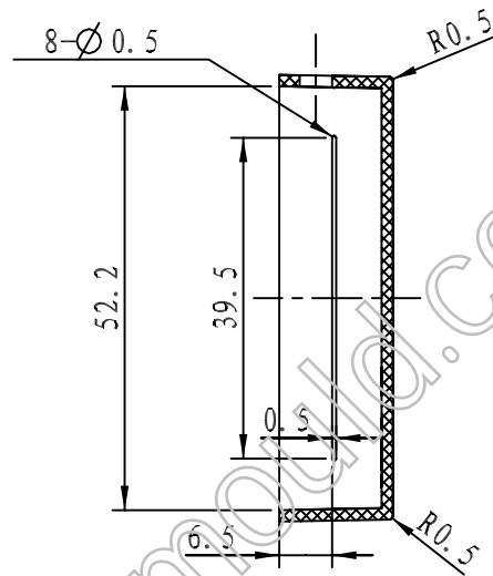
剖面 A-A
