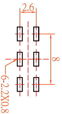
P.C.B.LAYOUT
