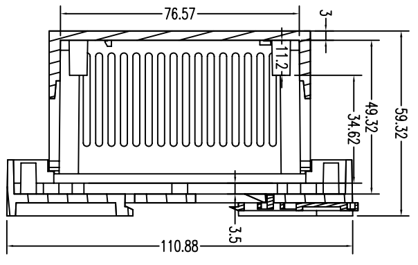
剖面 A-A
