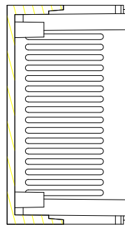
剖面 A-A
