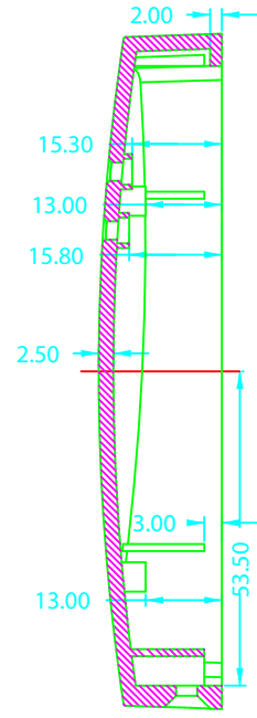
SECTION A-A
