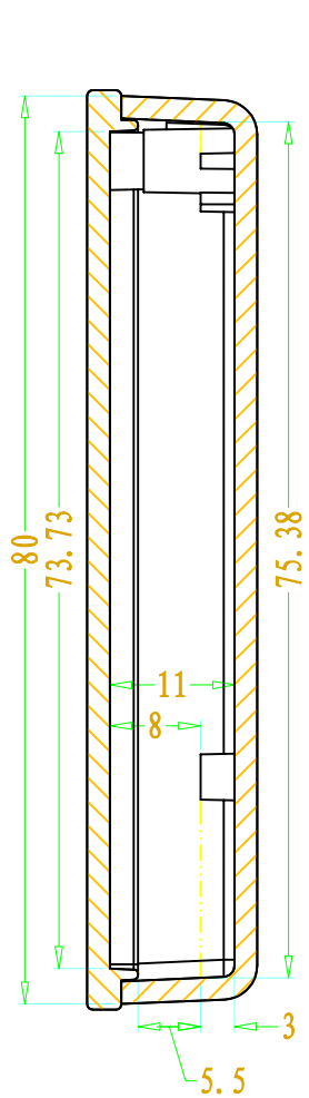
SEC A-A
