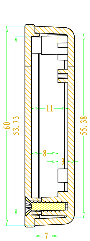
SEC A-A
