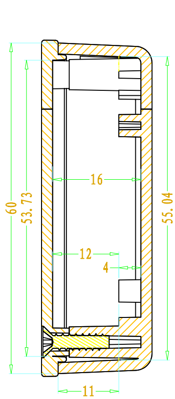
SEC A-A
