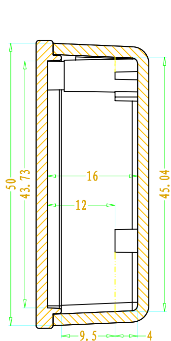
SEC A-A
