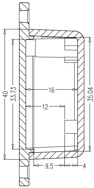
SEC A-A
