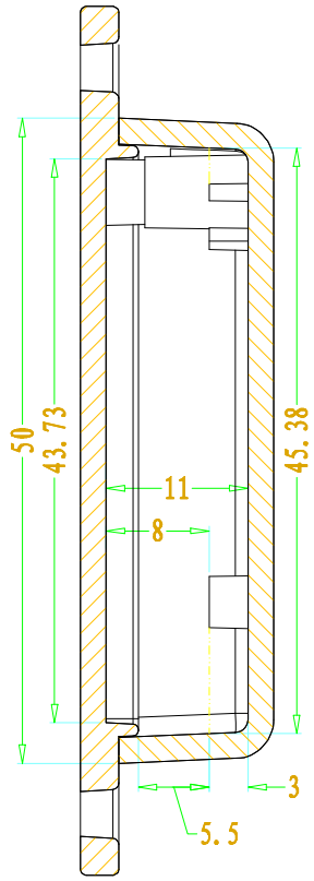
SEC A-A
