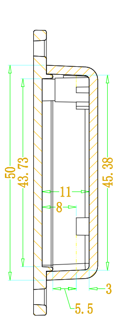
SEC A-A
