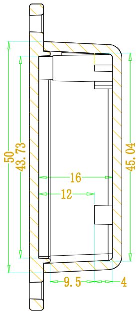
SEC A-A
