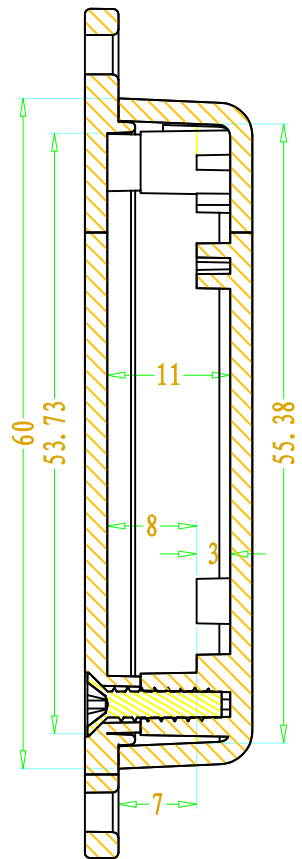
SEC A-A
